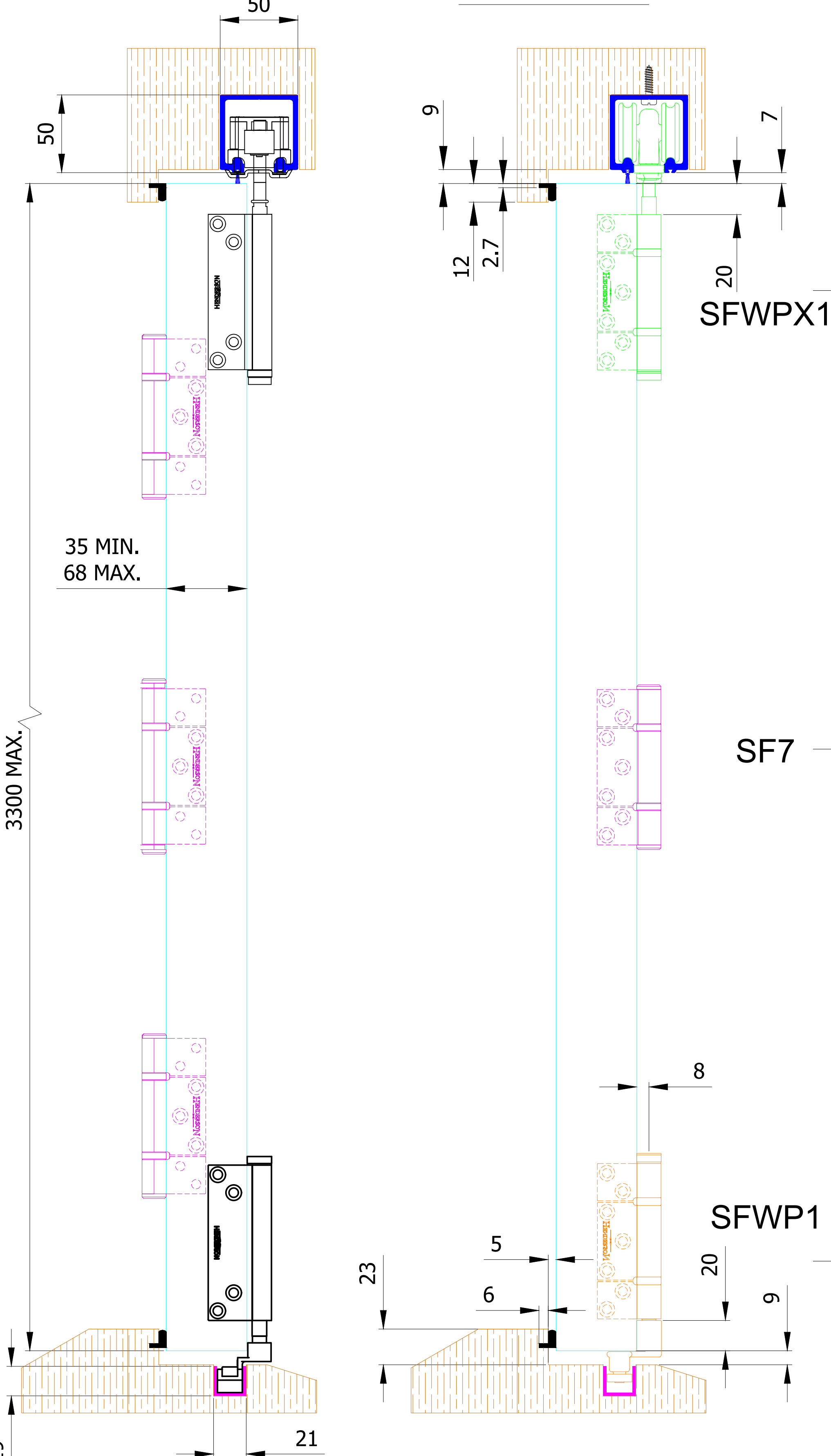
SECTION A-A
